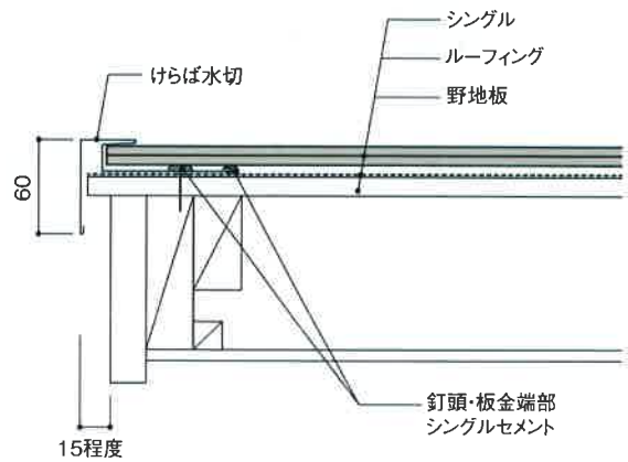
のぼり木無タイプ仕上げ
