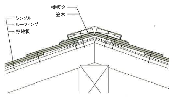
大棟板金仕上げ
