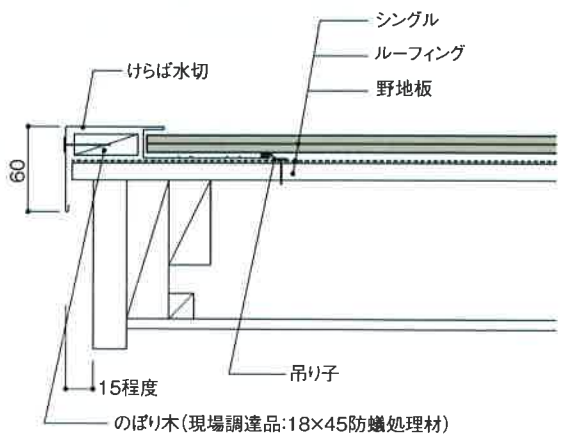
のぼり木タイプ仕上げ
