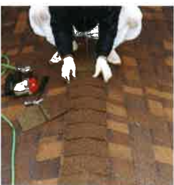
ヒップアンドリッジ取付け
