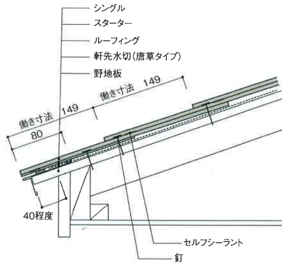
唐草タイプ水切仕上げ
