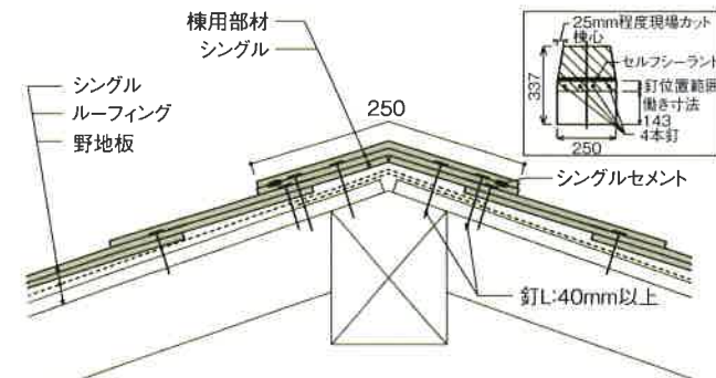
隅棟同質仕上げ
