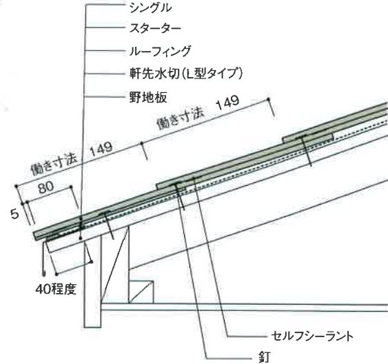
L型タイプ水切仕上げ
