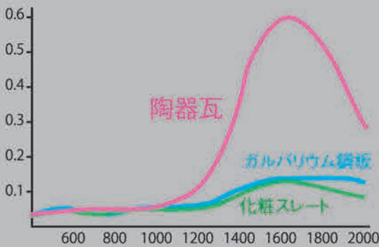
屋根材の違いによる騒音の吸音率
